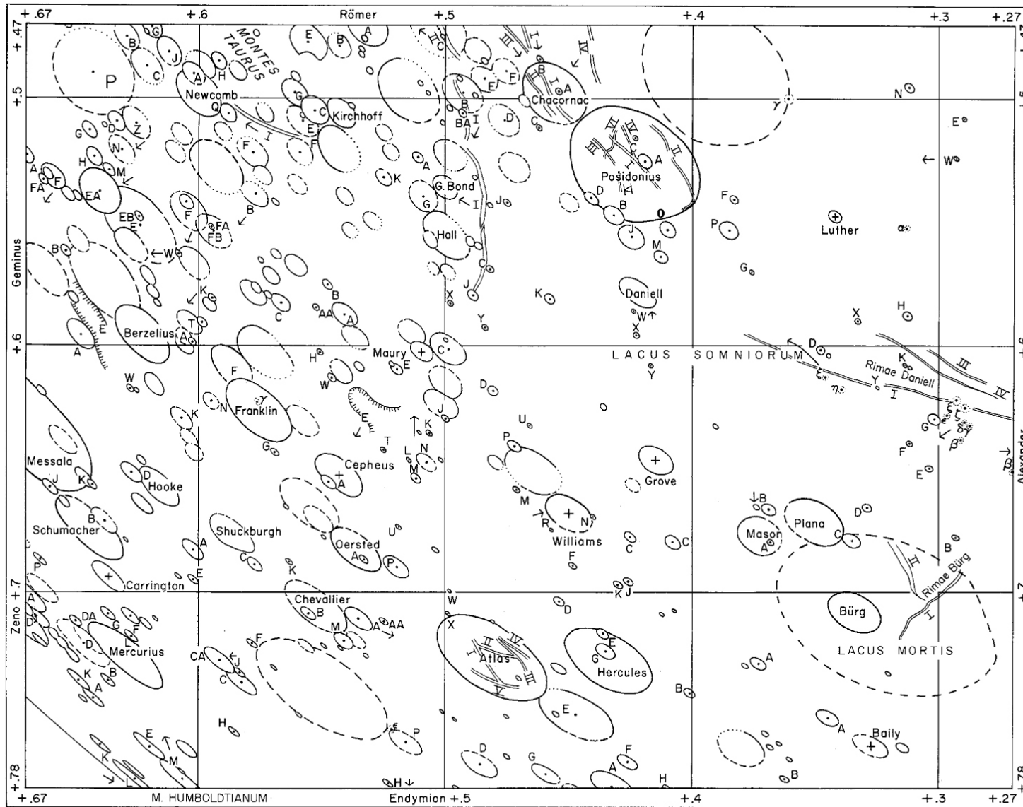
LUNAR NOMENCLATURE
