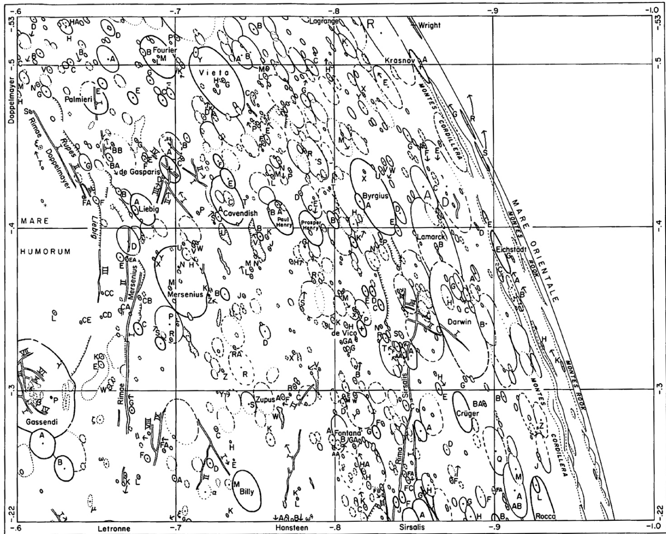
LUNAR NOMENCLATURE
