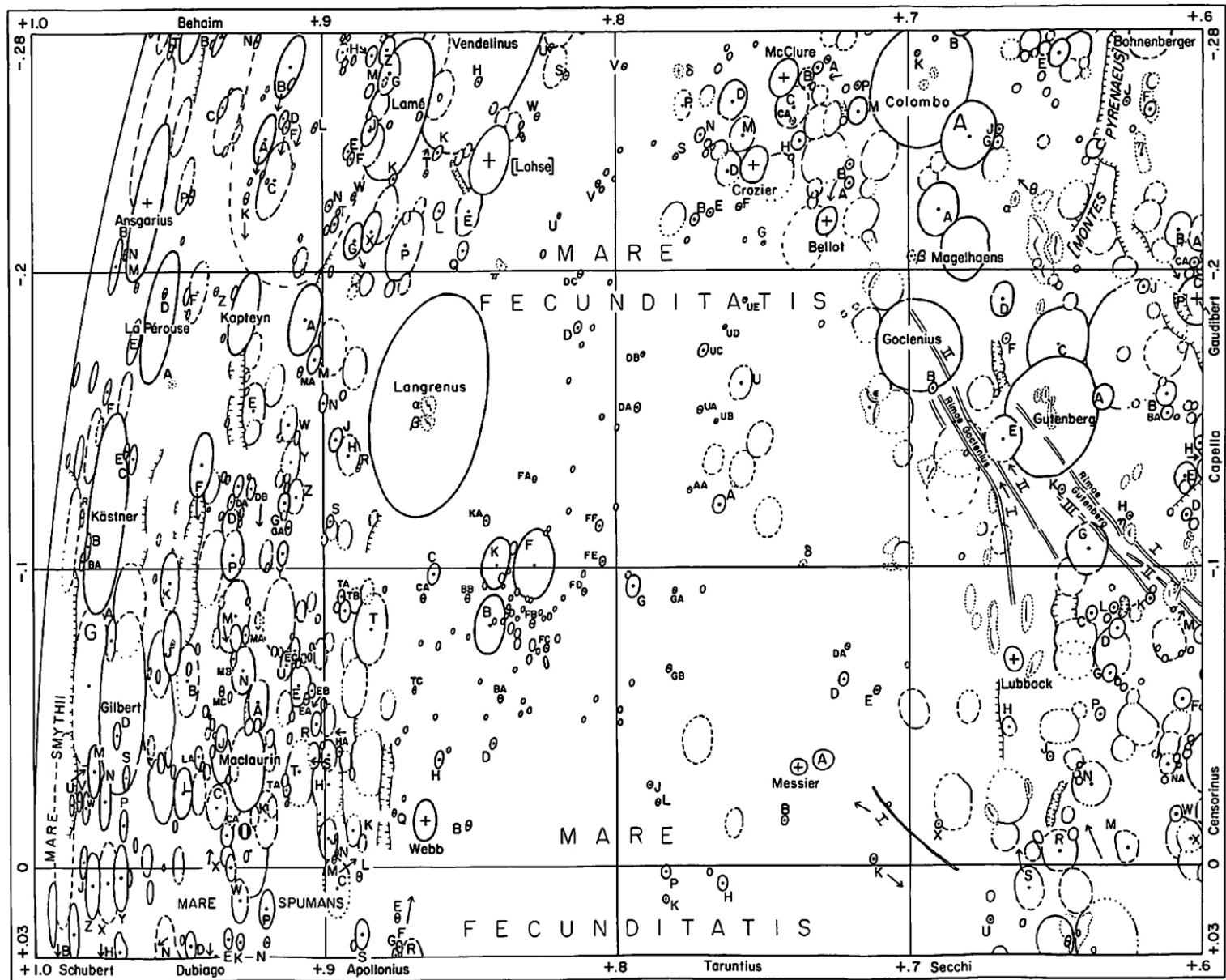
LUNAR NOMENCLATURE
