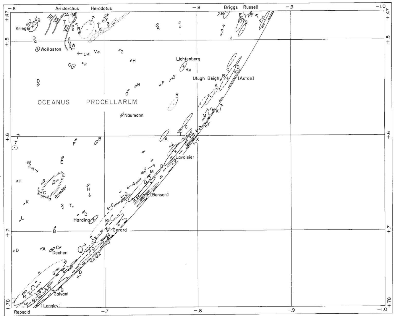
LUNAR NOMENCLATURE
