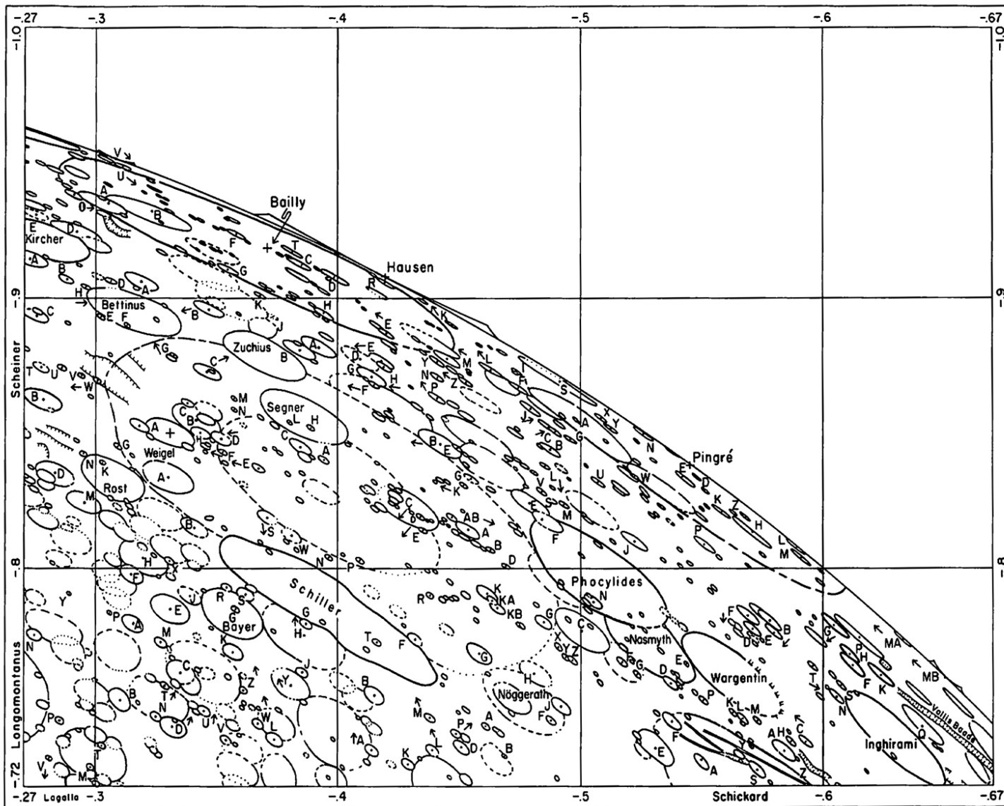
LUNAR NOMENCLATURE
