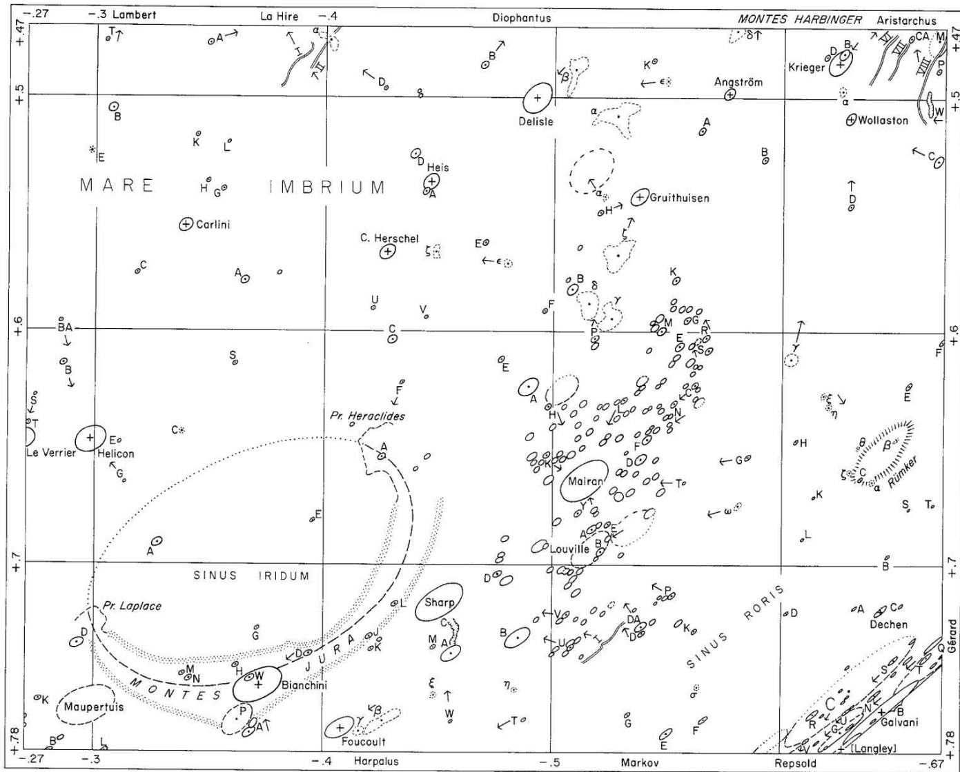
LUNAR NOMENCLATURE
