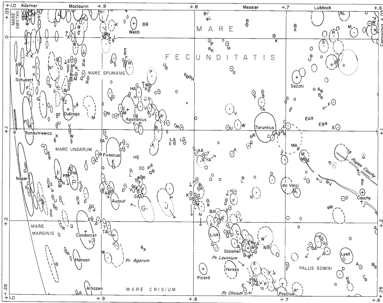
LUNAR NOMENCLATURE
