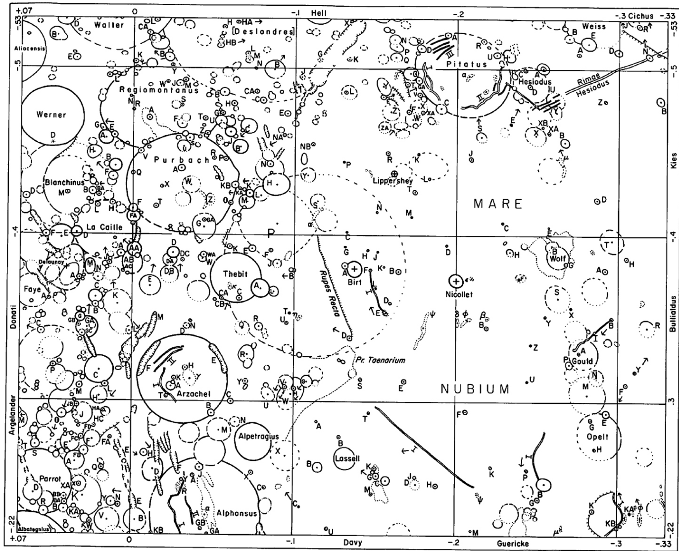
LUNAR NOMENCLATURE
