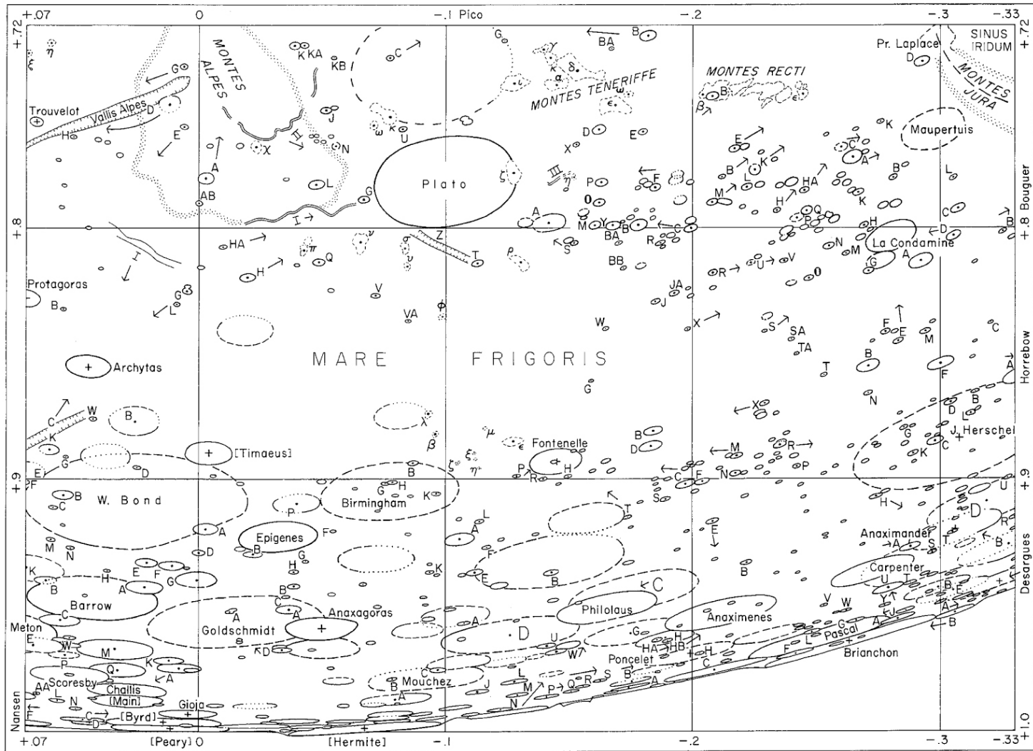
LUNAR NOMENCLATURE
